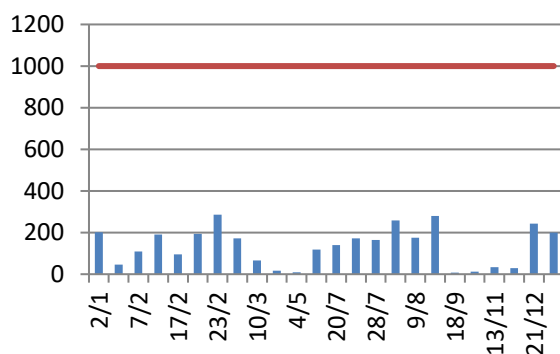
Charge entrante DBO5 en kg/j
